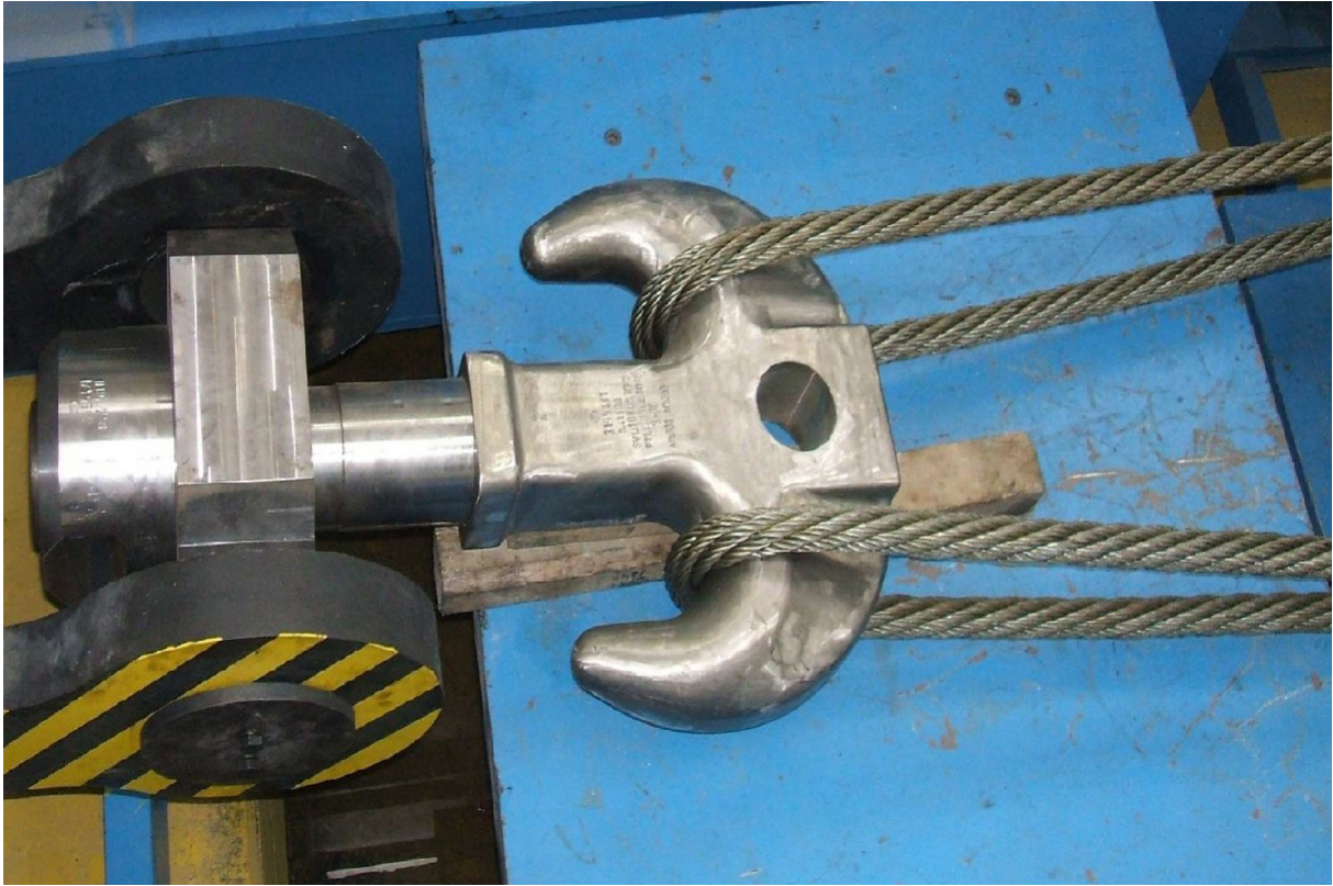
Het testen van een hijshaak op de grote testbank bij Irizar Forge Ltd. In Spanje
